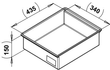
Medidas internas em mm da gaveta refil linha 400
