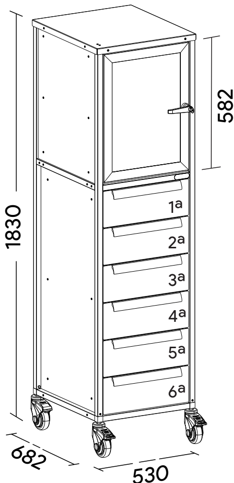
Dimensões do Armário
