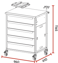
Suporte para caixa de perfuro cortante de 7L
